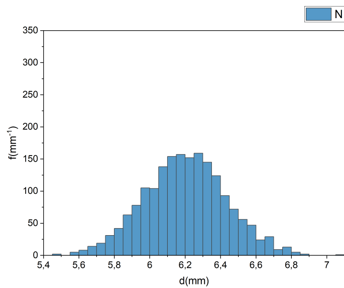
Obrázek 2: Histogram se šířkou binu 0,05 mm
