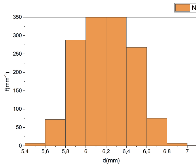
Obrázek 3: Histogram se šířkou binu 0,2 mm
