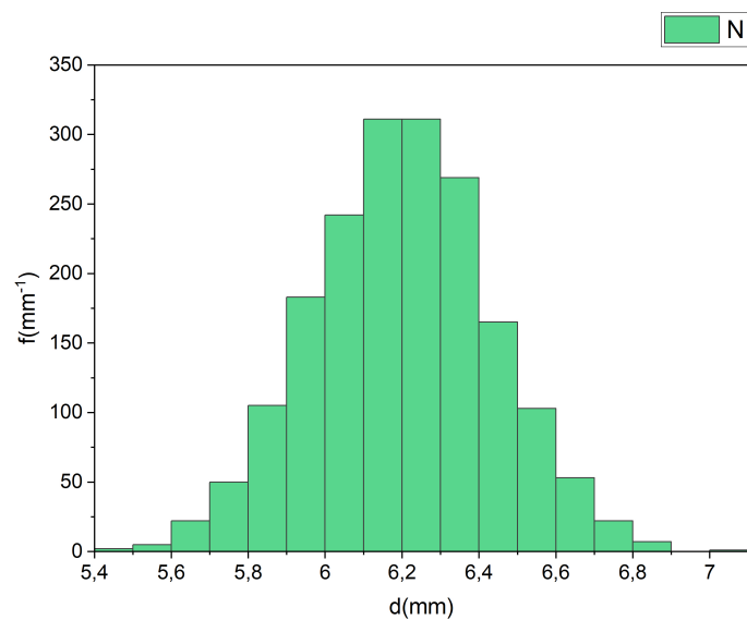
Obrázek 1: Histogram s automatickou šířkou binu (0,1 mm)
